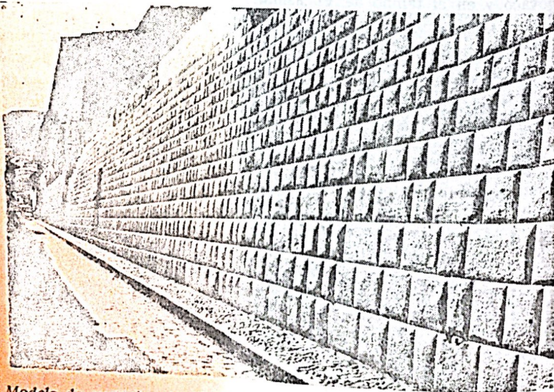
Modelo de cantería y construcción inca en "degradé". Muro de la calle Loreto en el Cusco.
